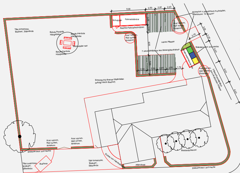
ENTWURF FREIANLAGEN
